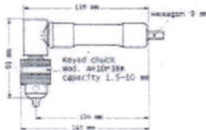
Mit 10mm Zahnkranz- Bohrfutter Typ: RADACK VPSFR 149,-
